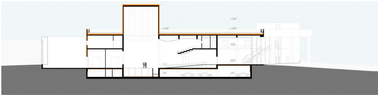
metszet M 1:250
